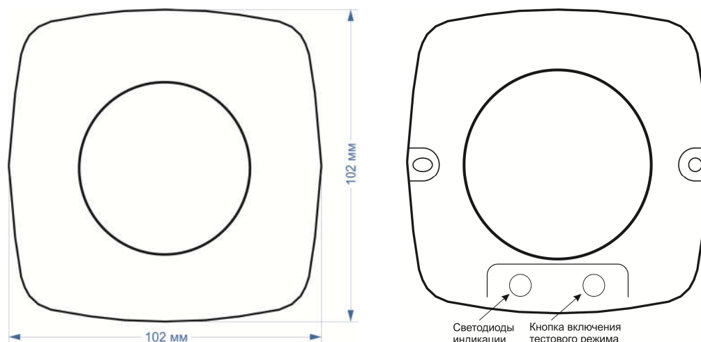
Рисунок 1. Внешний вид датчика. Габаритные размеры при установленной крышке (слева). Расположение элементов управления при снятой крышке (справа)
